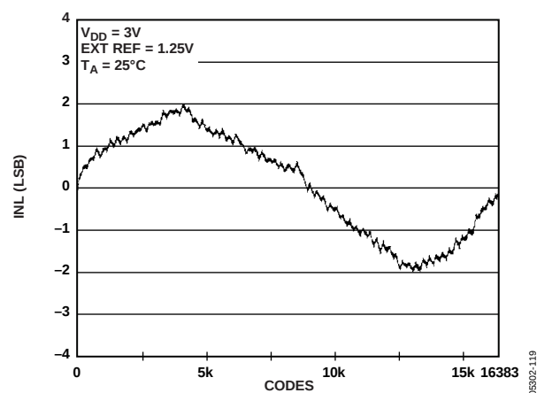
Figure 20. INL AD5648-1
