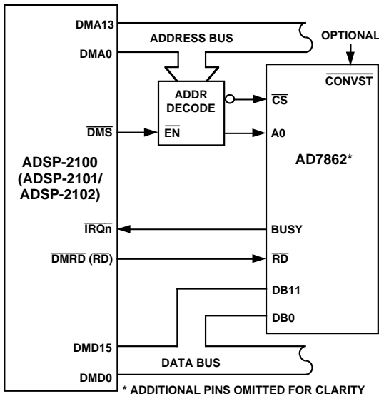
Figure 14. AD7862–ADSP-2100 Interface
