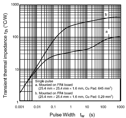
Fig. 7.12 r_{th} - t_w
