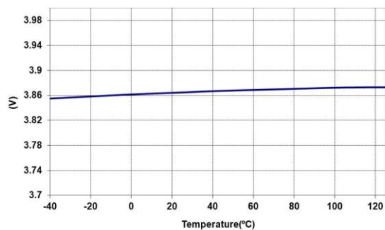
Vcc_UVLO_Stop
