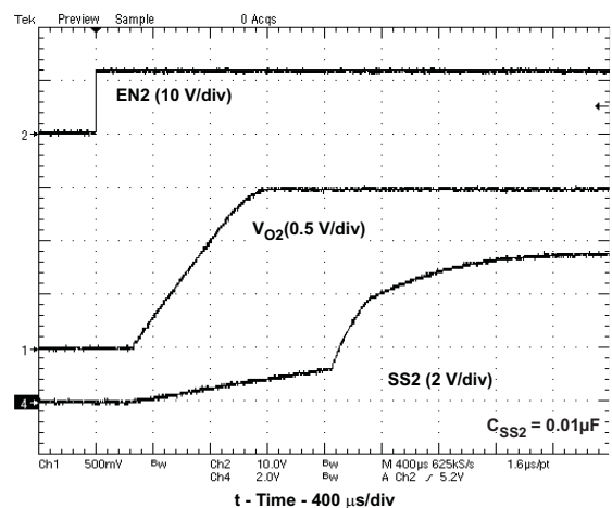
Figure 11. \text{VO2}=1.5\text{V} , SoftStart
