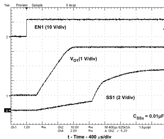
Figure 10. \text{VO1}=3.3\text{V} , SoftStart
